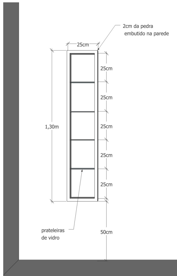
Vista 01 - Nicho semi embutido com medidas
