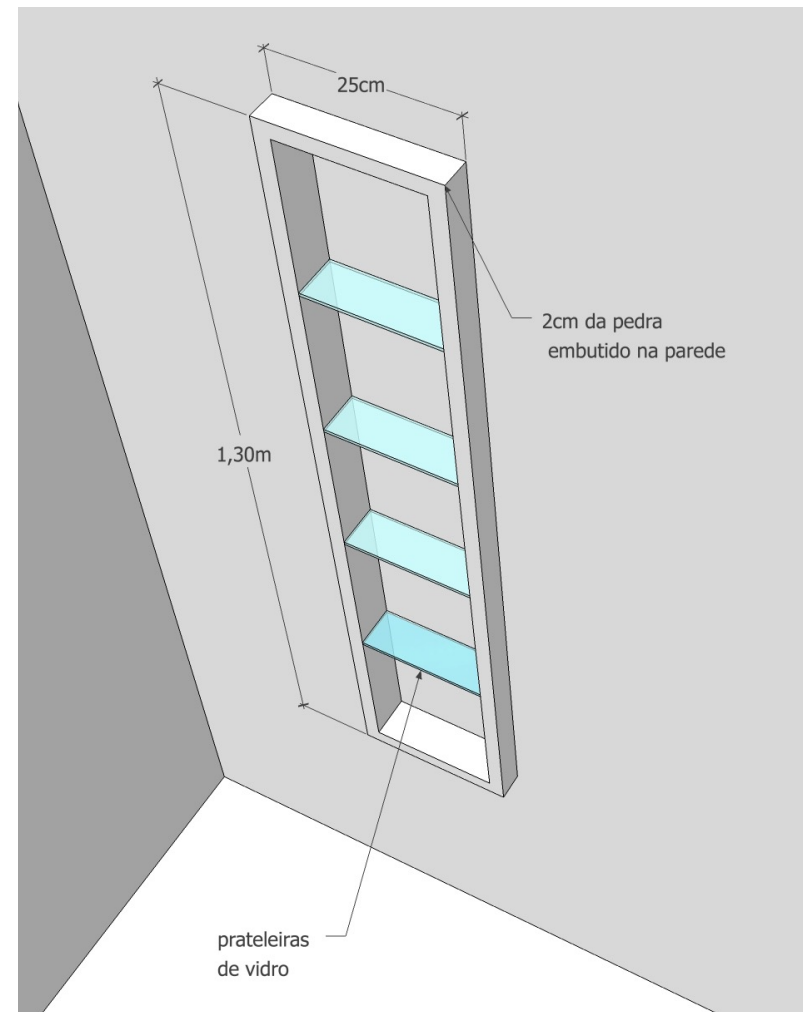
Vista 02 - Nicho semi embutido com medidas
